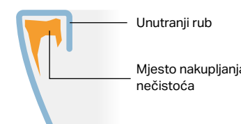
Klasična WC školjka s rubom za ispiranje
