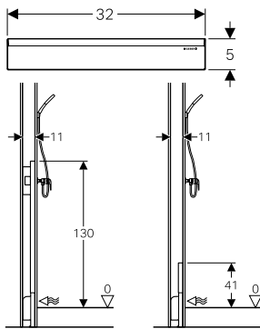
Geberit zidni tuš sifon
