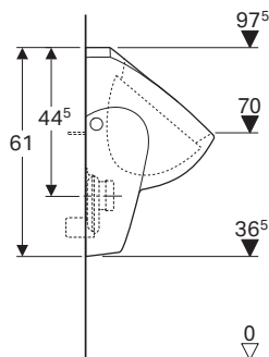
Geberit Alex pisoar, dovod odostraga, odvod prema natrag
