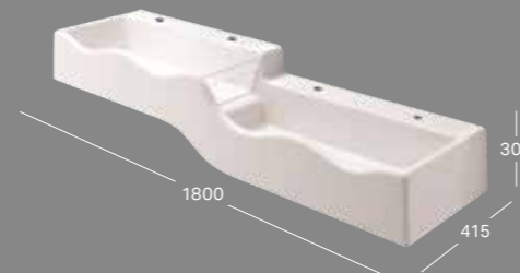
UMIVAONIK B 1800 / H 300 / T 415 za četiri armature, niže korito desno, materijal: Varicor® otvor za armaturu lijevo i desno, bez preljeva bez otvora za armaturu, bez preljeva
