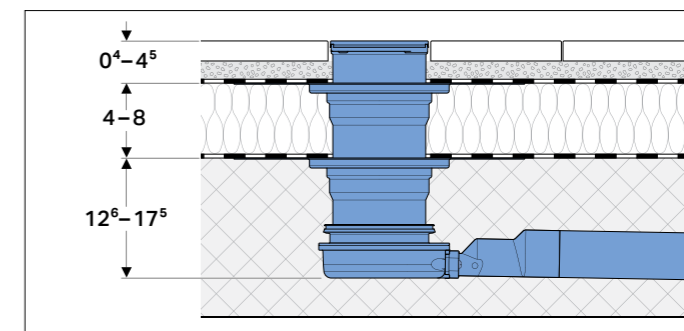
↑ Detalj spoja koji uključuje spoj na parnu branu, hidroizolaciju i podnu oblogu na podlozi od sitnog granulata
