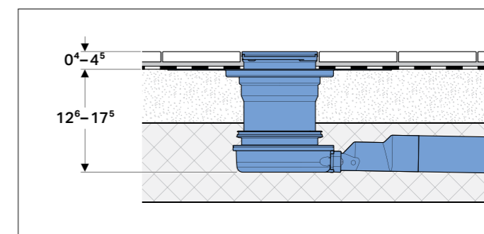
↑ Detalj spoja s prirubicom za hidroizolaciju na koti neposredno ispod podnih pločica
