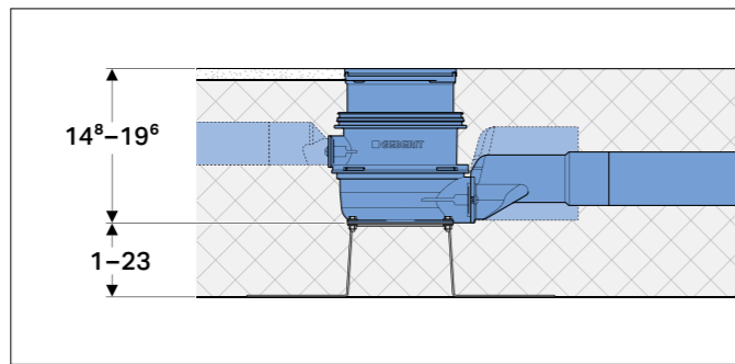
↑ Bez brtvljenja podnih površina ili armiranog betona
