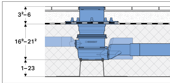
↑ Temeljna AB ploča s prirubničkim spojem na hidroizolaciju
