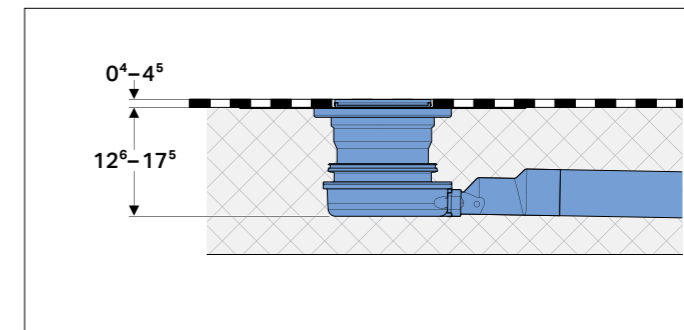
↑ Detalj hidroizolacijskog premaza s prirubicom od nehrđajućeg čelika
