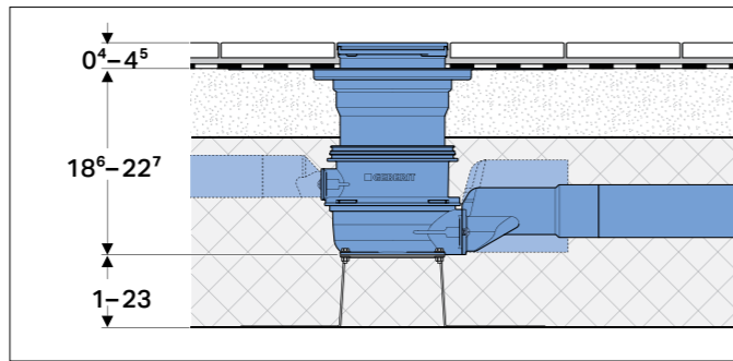
↑ Ploče u kombinaciji s prirubnicom od nehrđajućeg čelika
